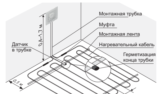
Рисунок 1. Монтаж терморегулятора и системы «теплый пол»
